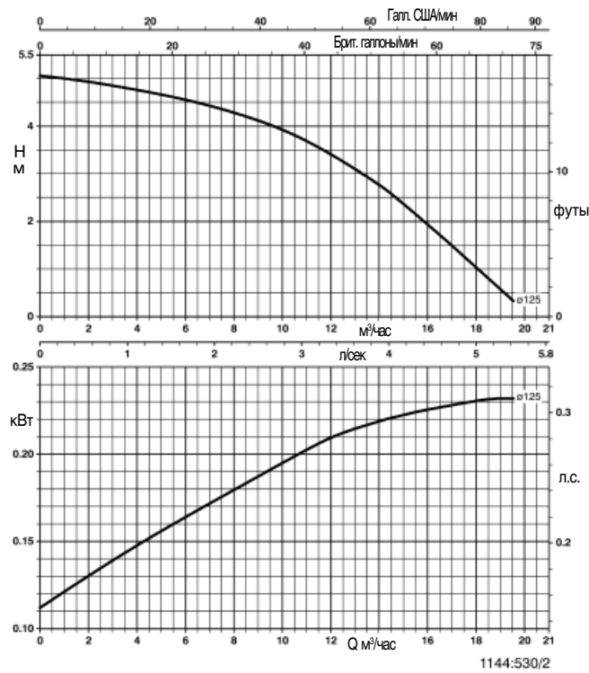
Trialine Z 40-125/024
