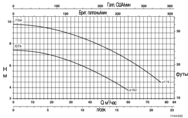
Trialine Z 65-160
