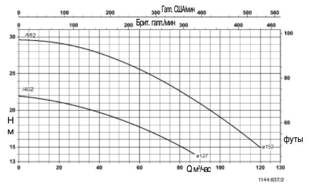
Trialine Z 65-160
